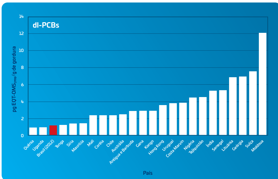
Figura 32: Níveis médios de dioxin-like PCB (A) e PCB indicadores (B) em leite materno no Brasil em 2012 em comparação com os resultados de outros países no período de 2008/2009.
