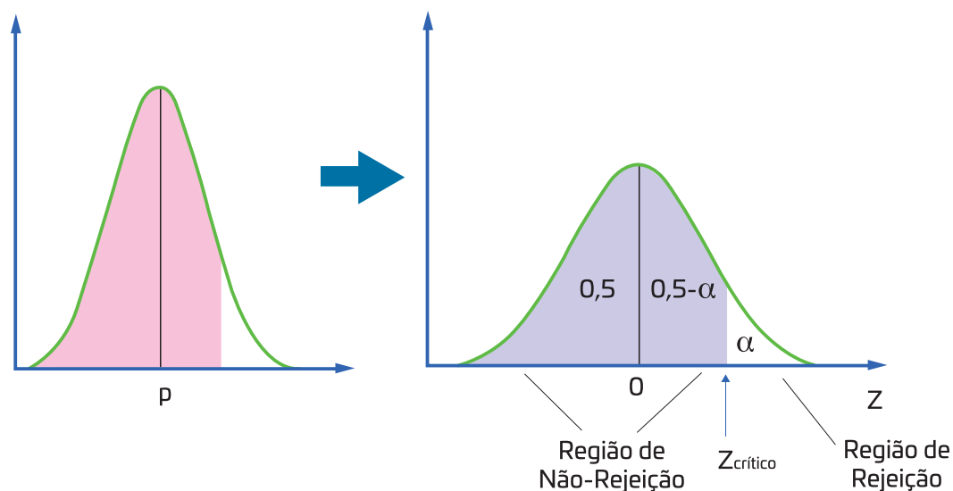
Figura 28: Teste z de hipóteses para proporção, unicaudal, com nível de confiança (1-\alpha)
