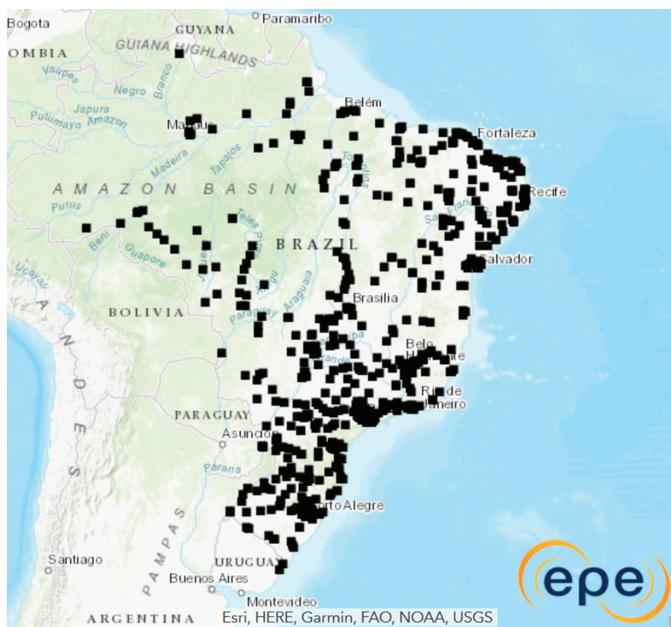
Figura 23: Subestações existentes no Brasil
